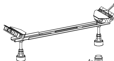
据付用脚参考図 (Non Scale)
